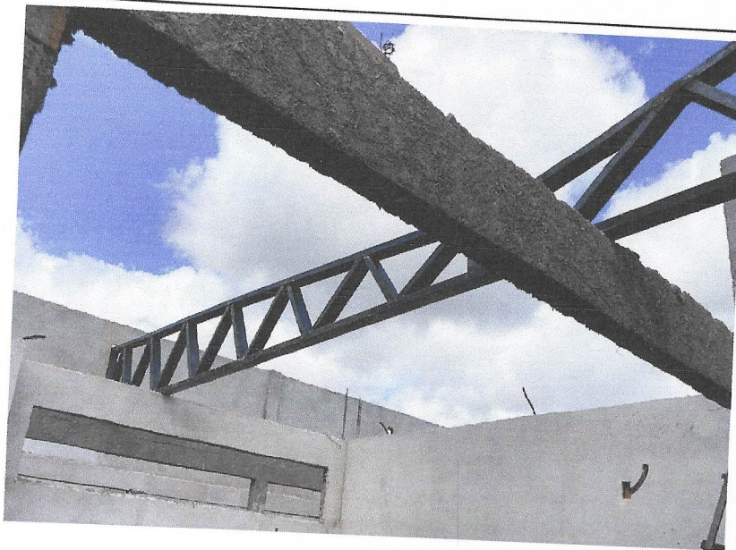
FOTO 64: ESTRUTURA METÁLICA DA COBERTURA
